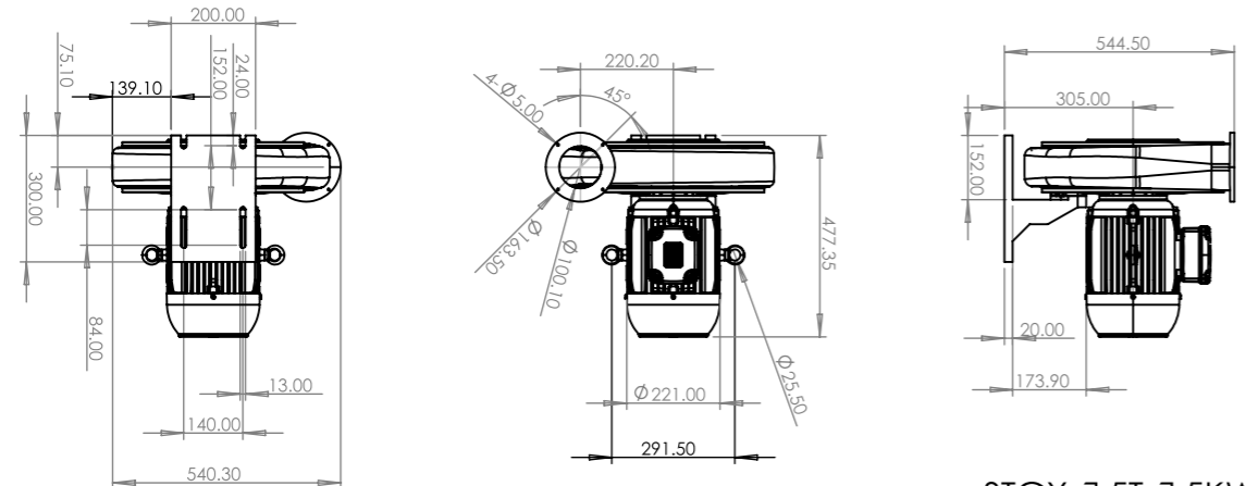
STGY-7.5T-7.5KW 具体需求型号请联系客服人员
