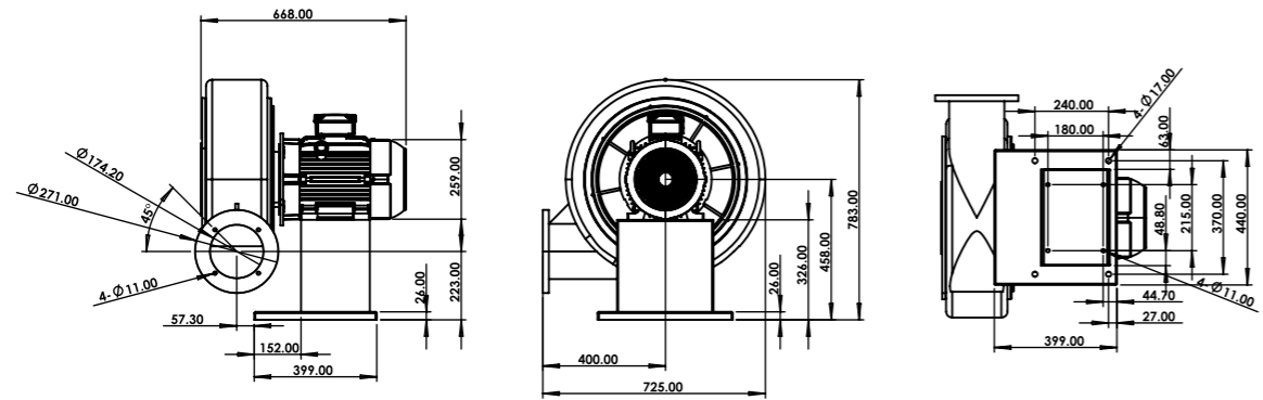
STGY-15T-15KW 具体需求型号请联系客服人员
